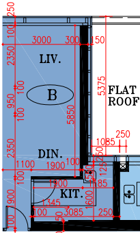
Part Plan of Flat B of 67/F. of Zone 1 of Tower 20* 第20座，第1區，67樓B室部分平面圖*
