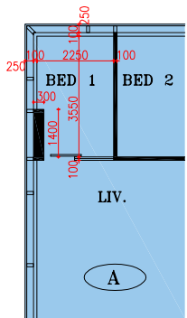
Part Plan of Flat A of 67/F. of Zone 1 of Tower 20* 第20座，第1區，67樓A室部分平面圖*
