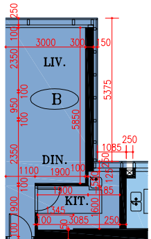
Part Plan of Flat B of 68/F. of Zone 1 of Tower 20* 第20座，第1區，68樓B室部分平面圖*
