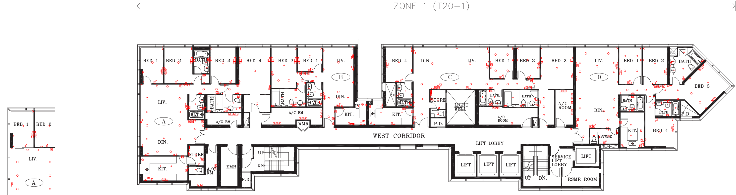
Part Plan of Flat A of 86/F. of Zone 1 of Tower 20* 第20座，第1區，86樓A室部分平面圖*
