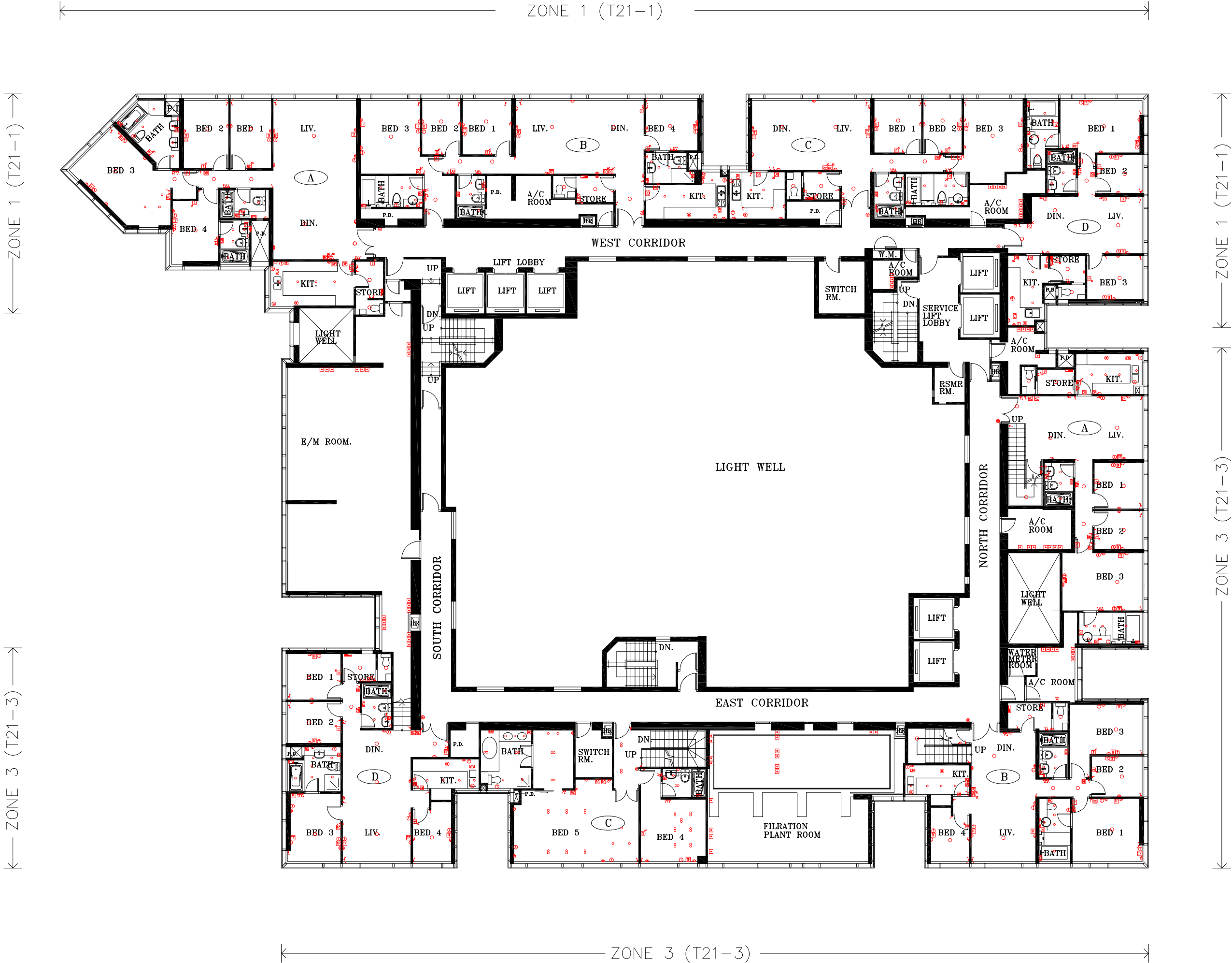
Part Plan of Flat C of 81/F. of Zone 3 of Tower 21* 第21座，第3區，81樓C室部分平面圖*
