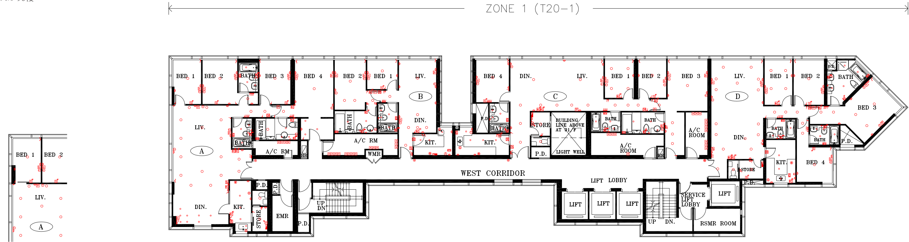
Part Plan of Flat A of 90/F. of Zone 1 of Tower 20* 第20座，第1區，90樓A室部分平面圖*
