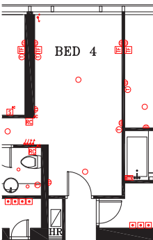
Part Plan of Flat A of 86/F. of Zone 1 of Tower 20* 第20座，第1區，86樓A室部分平面圖*
