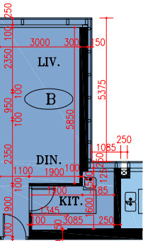
WEST CORRIDOR Part Plan of Flat B of 69/F. of Zone 1 of Tower 20* 第20座，第1區，69樓B室部分平面圖*
