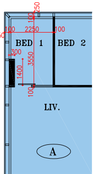
Part Plan of Flat A of 79/F. of Zone 1 of Tower 20* 第20座，第1區，79樓A室部分平面圖*
