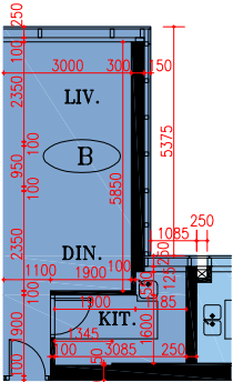
Part Plan of Flat B of 68/F. of Zone 1 of Tower 20* 第20座，第1區，68樓B室部分平面圖*
