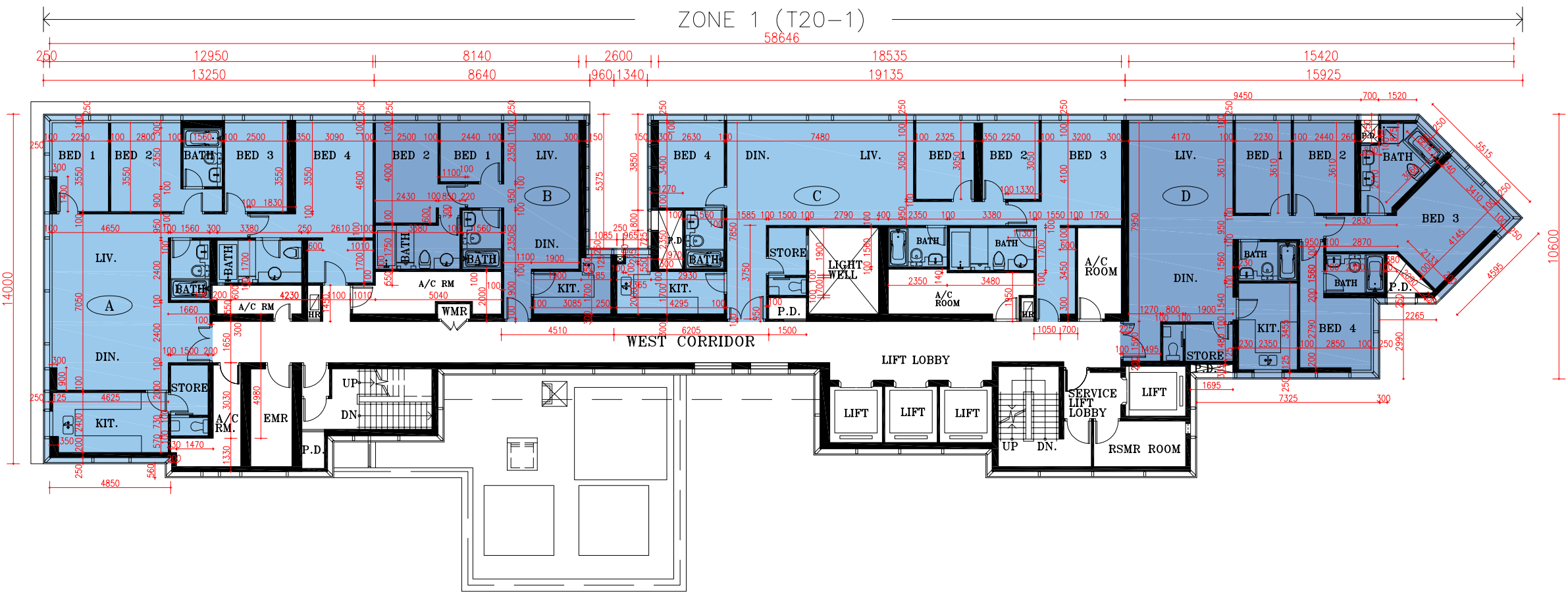
Part Plan of Flat A of 80/F. of Zone 1 of Tower 20* 第20座，第1區，80樓A室部分平面圖*
